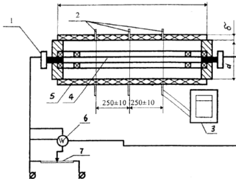
Рисунок 2. Принципиальная схема установки для определения теплопроводности материалов БОП-С:
